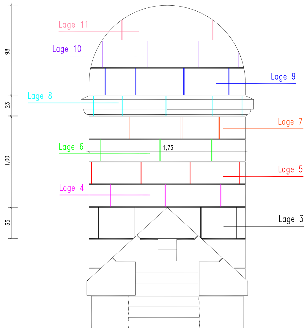
Systemschnitt Batardeau / Ansicht "Une Dame"
