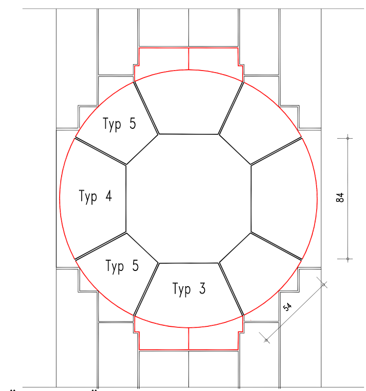
"Une Dame" Schichtengrundriss Lage 3
